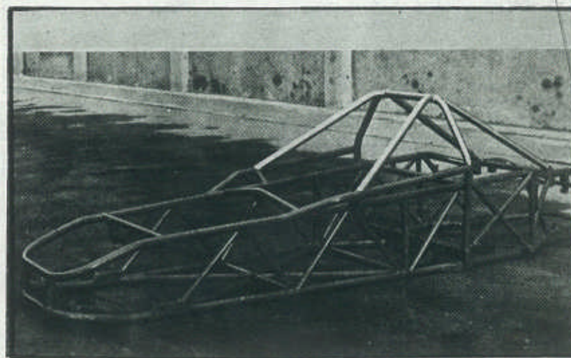
Aspecto de un chasis tubular para un monoplaza de autocross.
