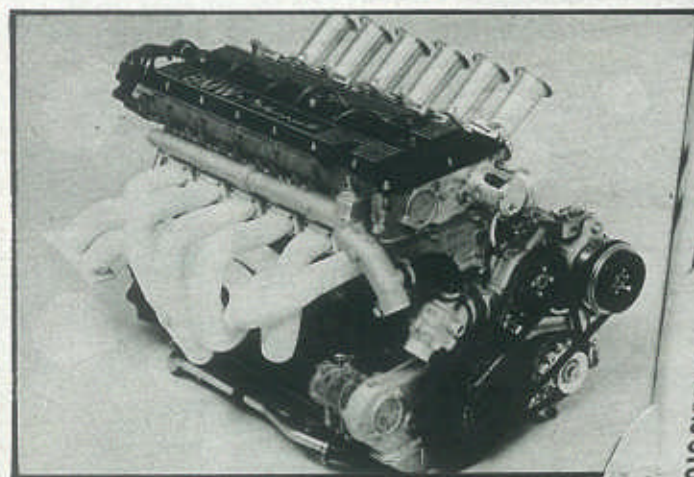
Aspecto del motor seis cilindros en línea de 3,5 litros, que desarrolla unos 480 CV.
