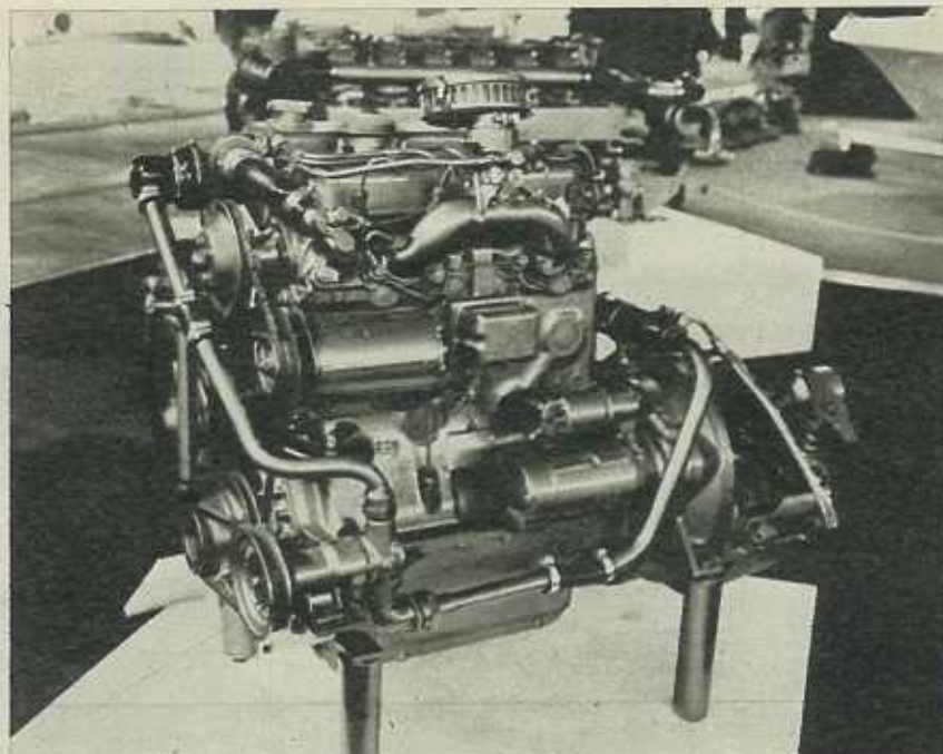
Motor Mercedes-Benz, construido por Mevosa (España) y marinizado en Inglaterra: su potencia es de 50 CV.
