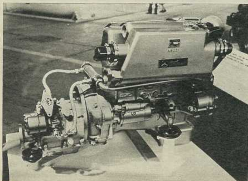
Motor Mercedes Benz (fabricación española) OM-636.
