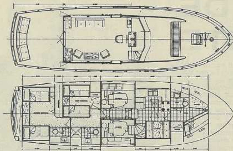
Hatteras 53 Motor Yacht. —Especificaciones. Eslora total: 16,18 metros; manga: 4,83 metros; calado: 1,22 metros; altura libre: 1,93 metros; capacidad agua potable: 1.000 litros; peso desplazamiento: 25 toneladas; grupo propulsor: dos motores diesel G. M.
