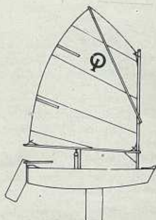
Eslora: 2,30 m. Manga: 1,13 m. Eslora en flotación: 2,15 m. Peso casco: 33 kg. Peso completo: 40 kg. Superficie velamen: 3,50 m 2 .
