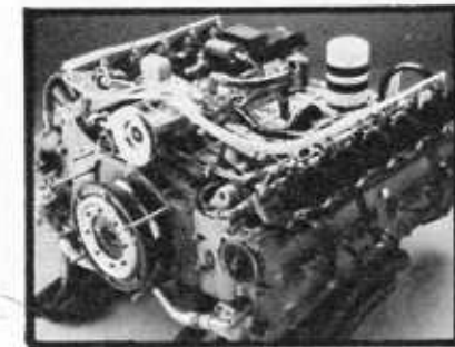
El motor 12 Boxer, campeón del mundo de resistencia, que lograría dos victorias en 1978 montado en el Brabham de Niki Lauda, empujando a Alfa a un retorno a la Fórmula 1.
