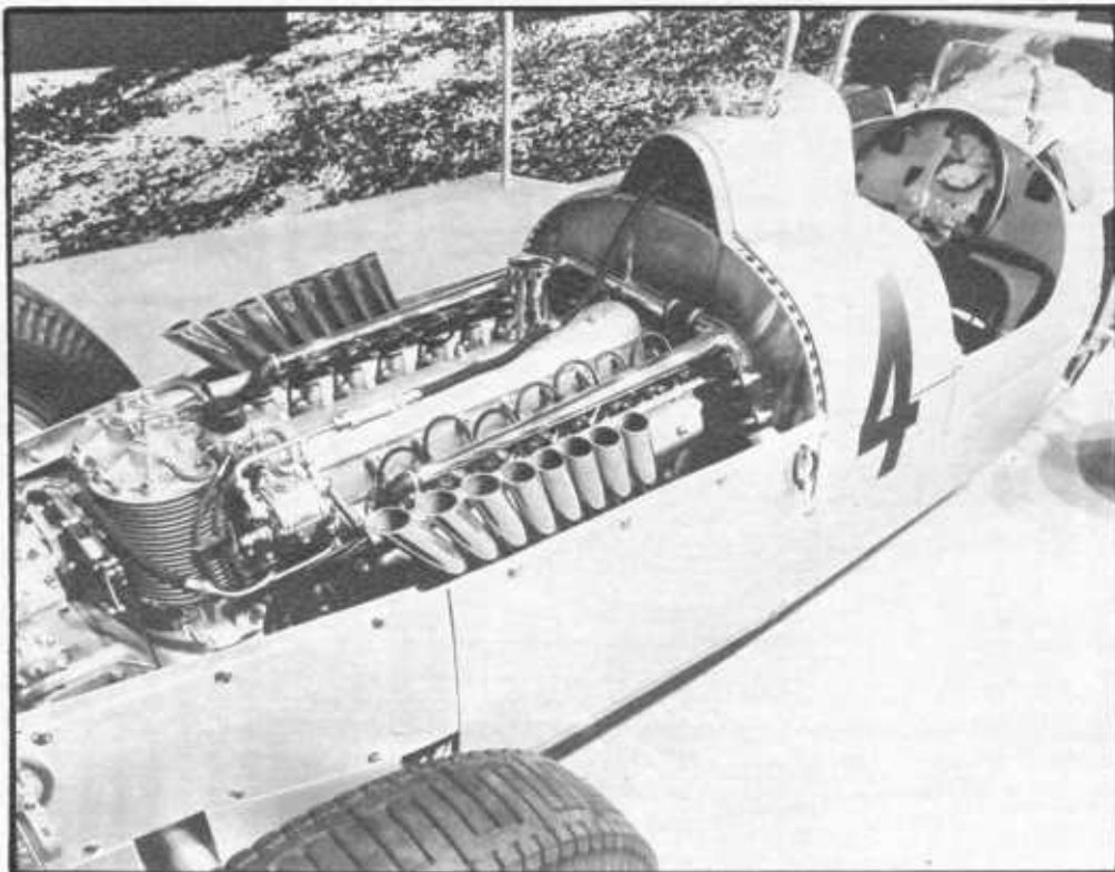
Aspecto del impresionante motor de 16 cilindros en V y más de seis litros de cilindrada, que desarrollaba 520 CV y lanzaba al coche a más de trescientos kilómetros por hora.
